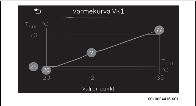
Bild 5 Utgångsvy värmekurva
